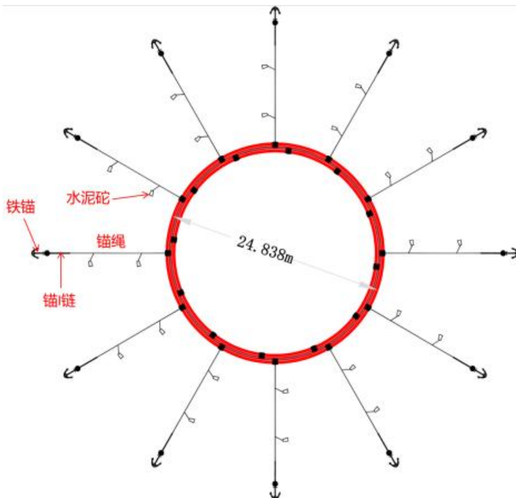
图 1.5.3-8 C90 圆形网箱锚固布置示意图
