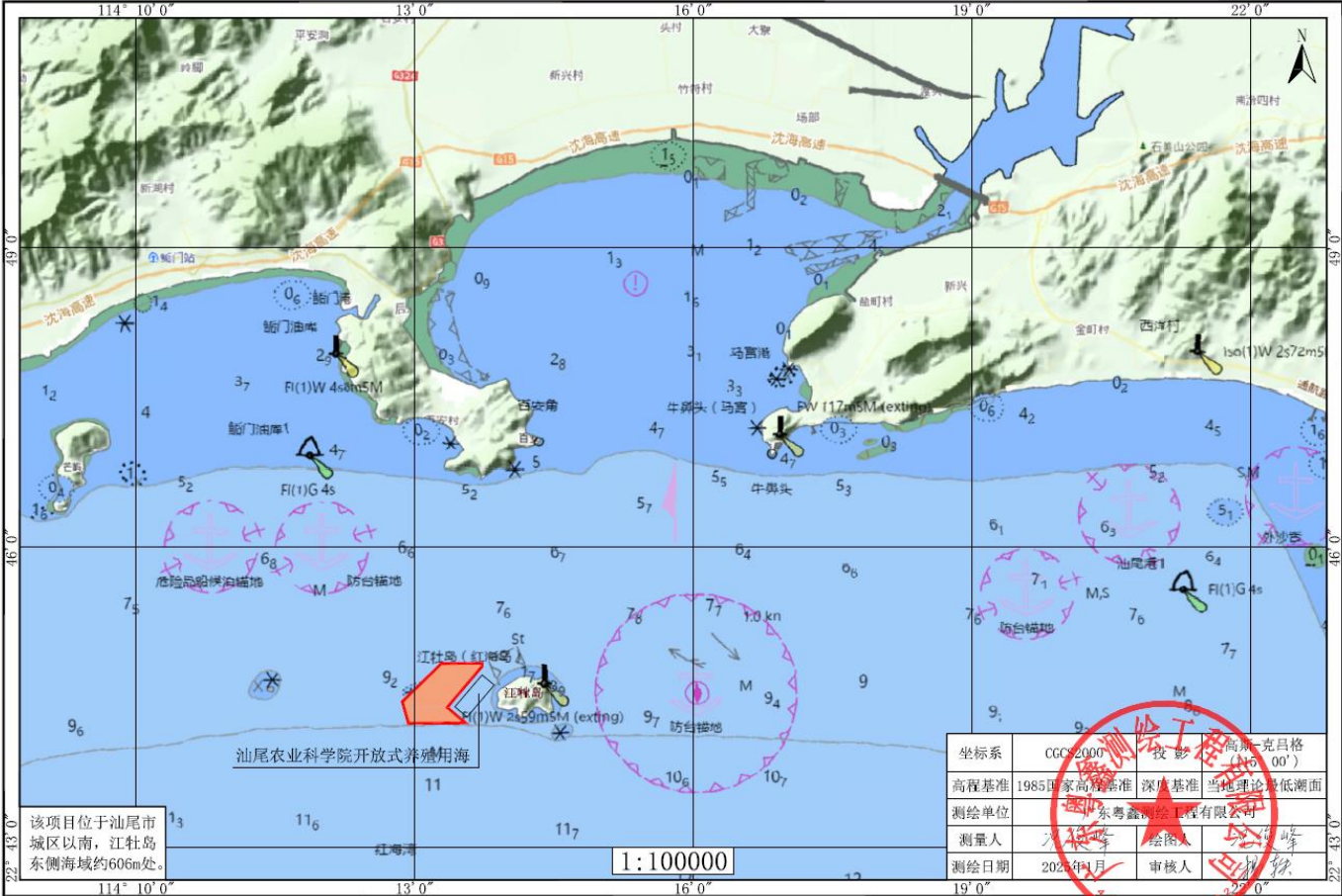
汕尾城区江牡岛西D区现代化海洋牧场开放式养殖用海项目宗海位置图
