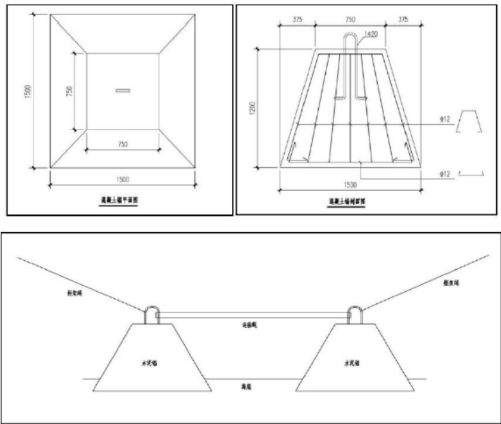
图 1.4.2-4 网箱固定混凝土锚示意图
