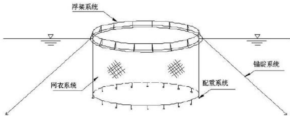
图 1.4.2-2 深水网箱结构示意图
