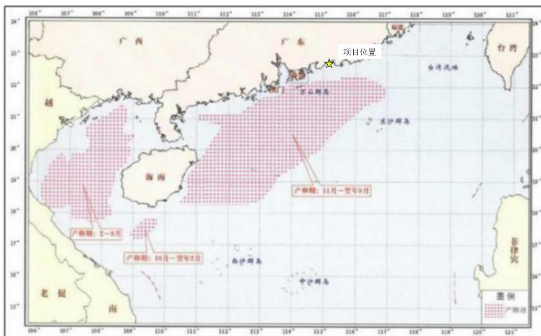
图 5.2.7-2 南海底层、近底层鱼类产卵场示意图
