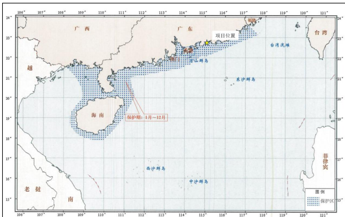
图 5.2.7-3 南海北部幼鱼繁育场保护区范围场示意图
