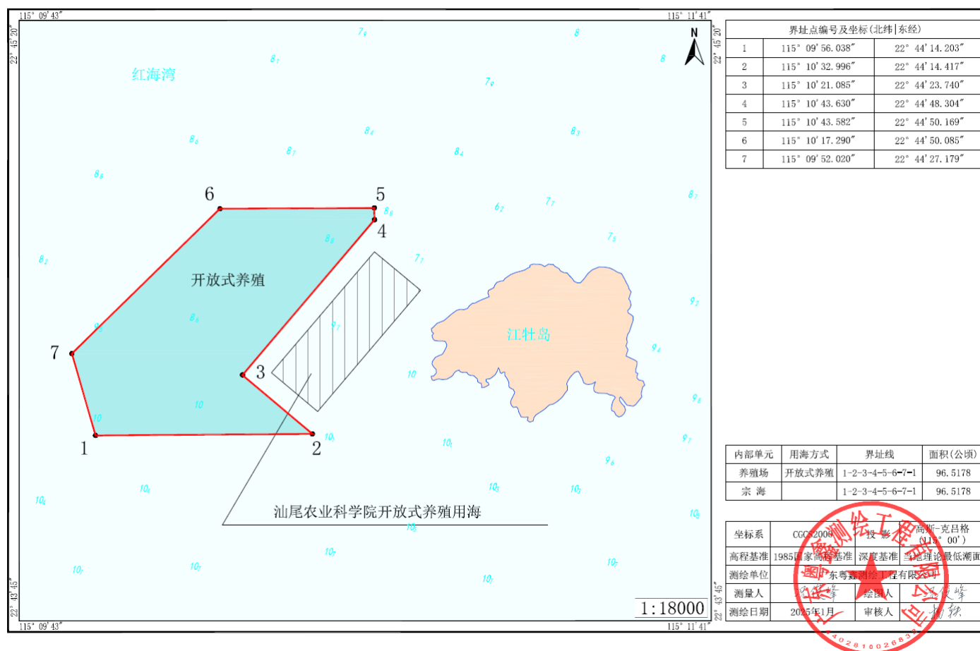
图 6.5-2 项目宗海界址图
