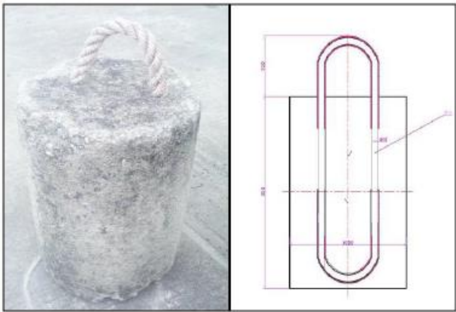
图 1.4.2-3 网衣坠子水泥沉块示意图
