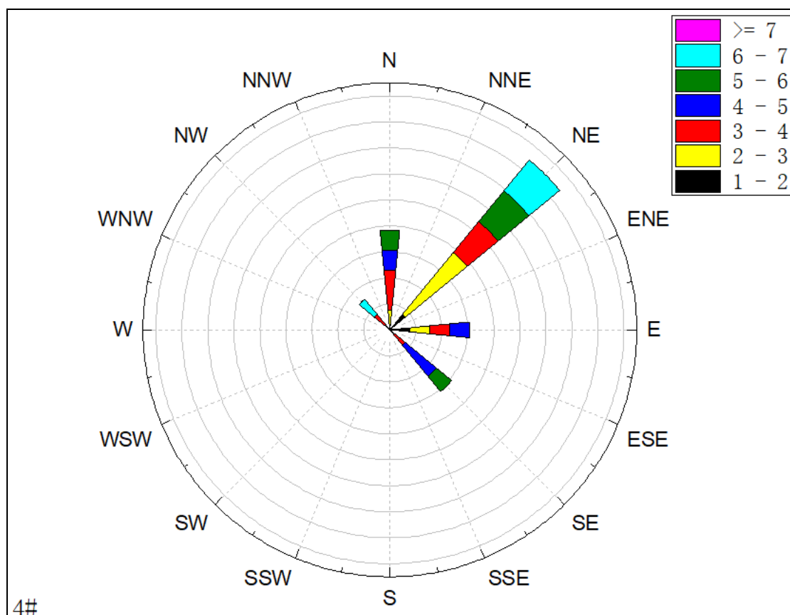
图 2.2.6-3 各垂线风玫瑰图
