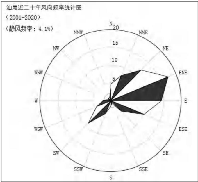
图 2.2.5-1 汕尾风向玫瑰图（静风频率 4.1%）
