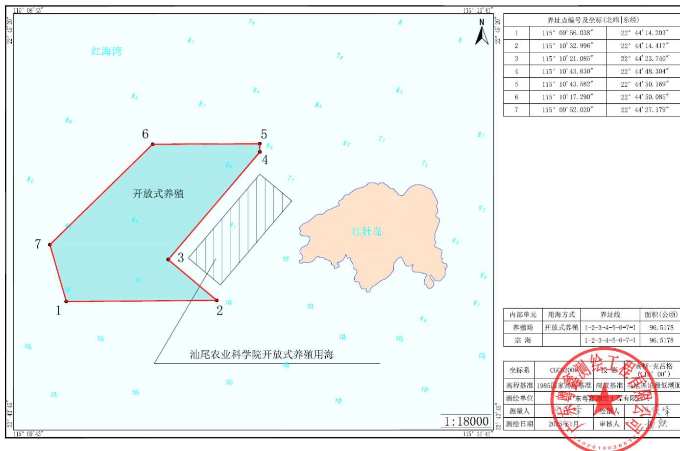
图 1.7-2 项目宗海界址图
